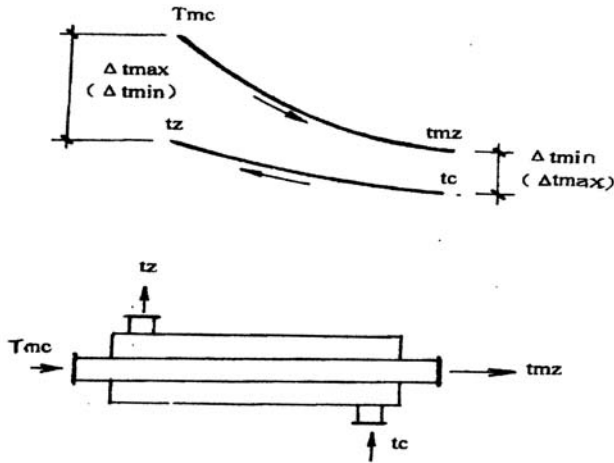
● 图 4 快速换热器水加热工况示意 ● \Delta t_{\max} = t_{mc} - t_z 或 \Delta t_{\max} = t_{mz} - t_c ● \Delta t_{\min} = t_{mz} - t_c 或 \Delta t_{\min} = t_{mc} - t_z
