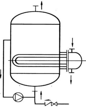
图 7 带外循环的容积式加热器
