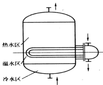
图 5 容积式加热器
