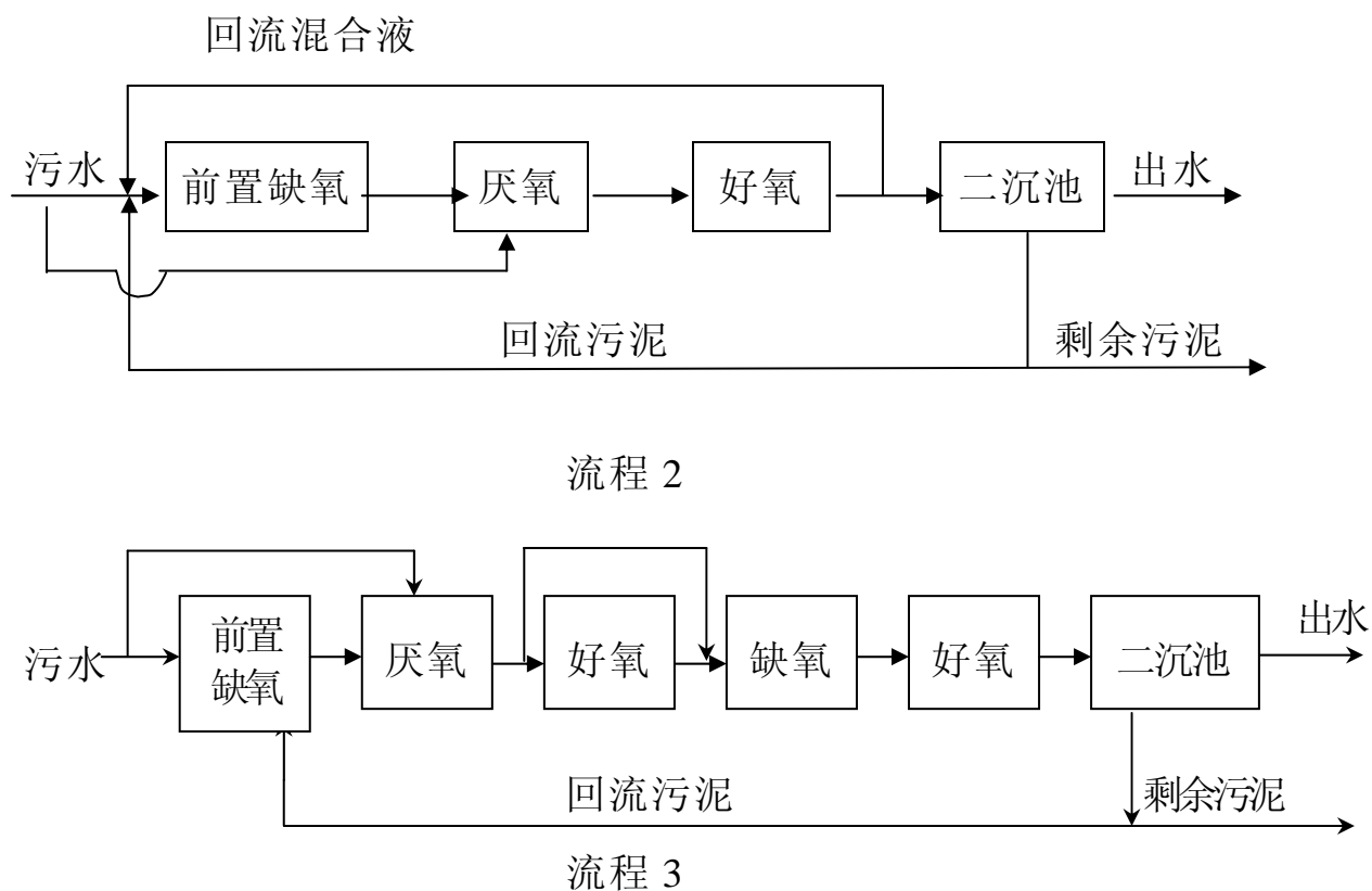
图 3 一些变型的工艺流程
